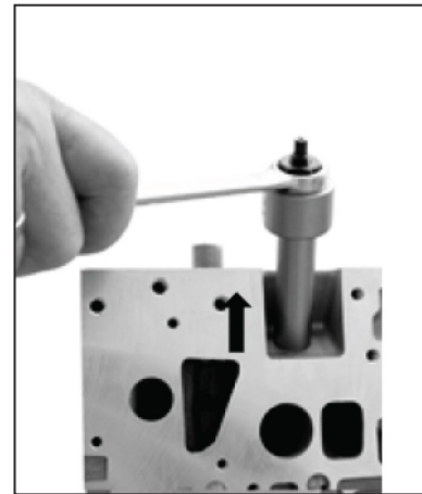
Uklonjen svjećasti grijač
